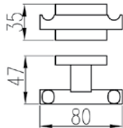
LovA Double Hook - Quadra BH022
